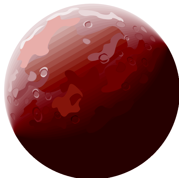
Mars
