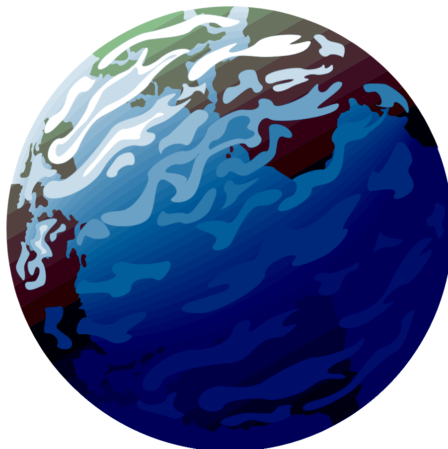
Earth
