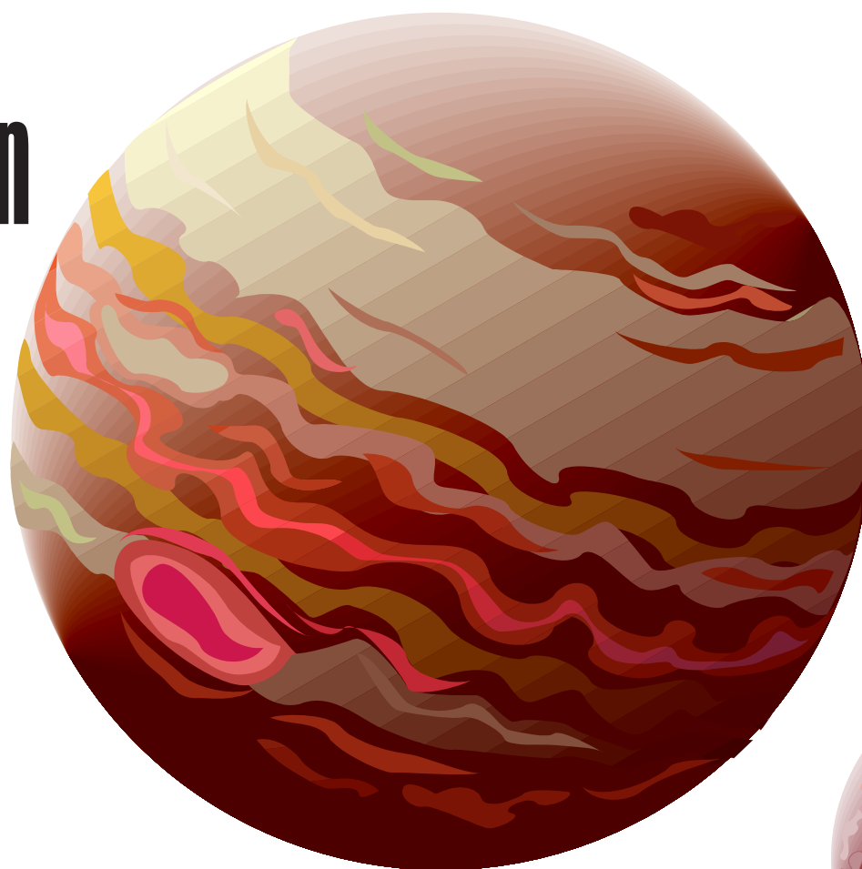
Uranus
