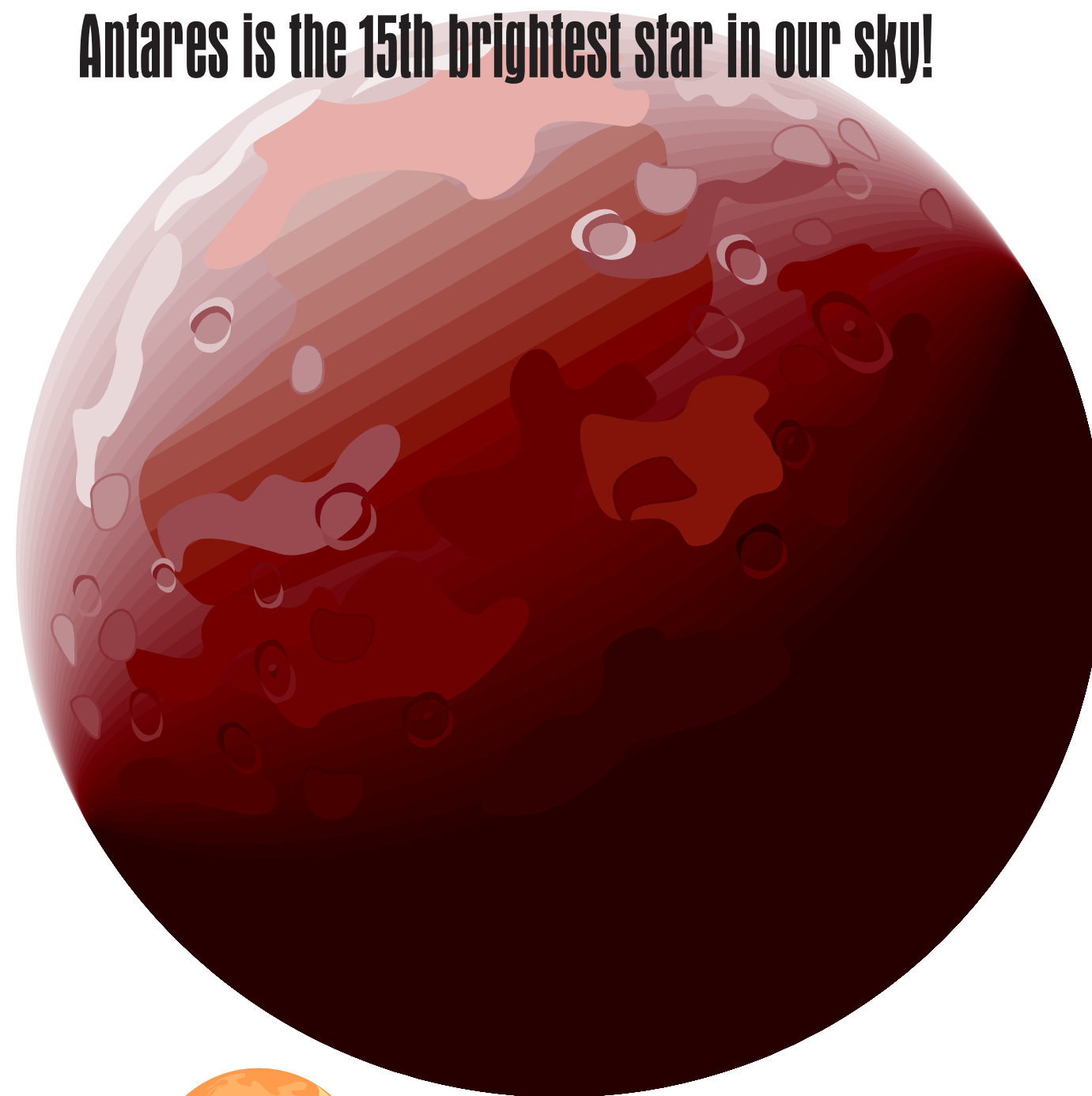
Antares
